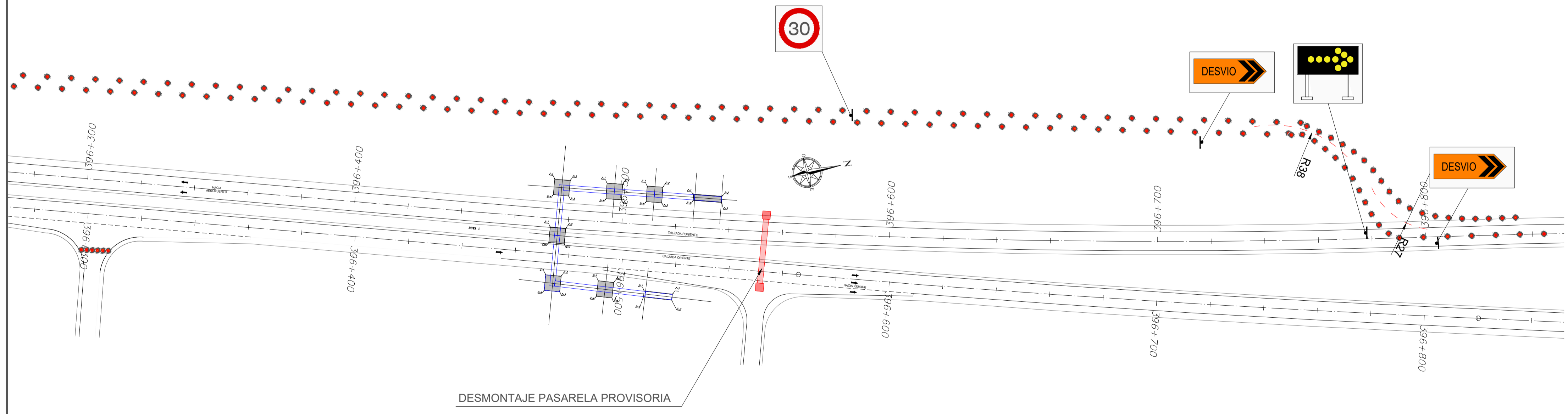
VISTA EN PLANTA ESCALA 1:1500
