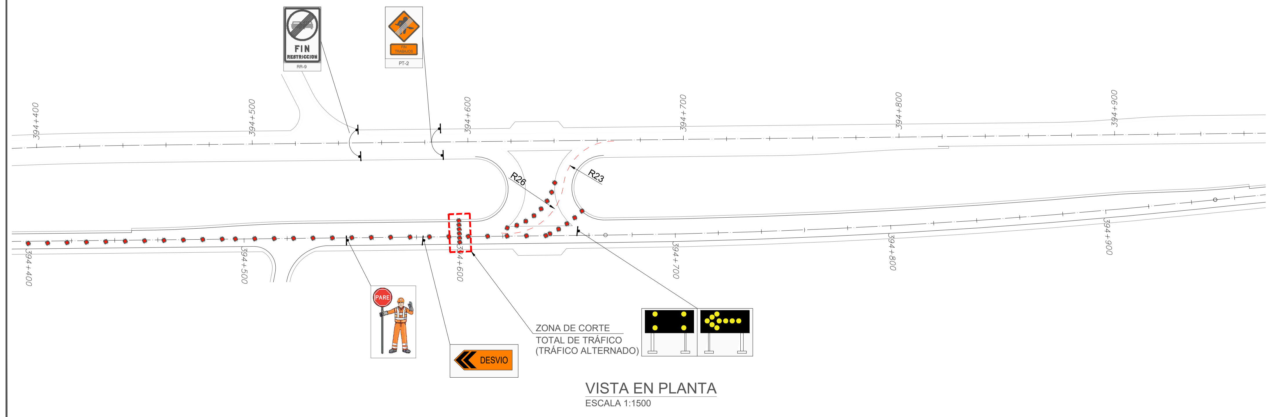
VISTA EN PLANTA ESCALA 1:1500
